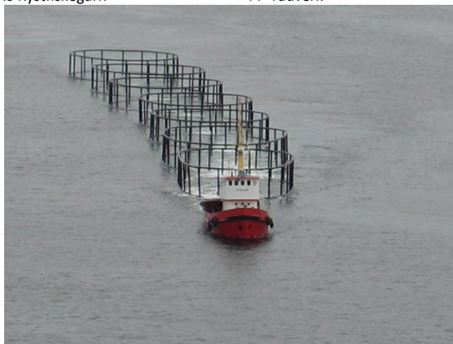
HDPE Flytekrager (Oppdrettsringer) og fuglenett
